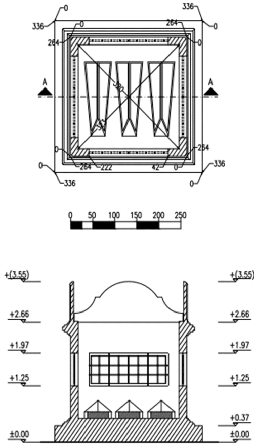
Şekil 1: Ahmed Kuddusi Mezar Anıtı röleve ve restitüsyon planı (Çizim: Humam Hamid).
